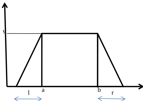
شکل ۱. عدد فازی دوزنقه‌ای
