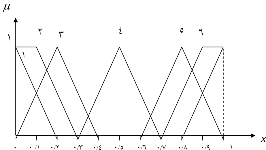
شکل ۲. اعداد فازی دوزنقه‌ای مربوطه به عبارتهای زبانی
