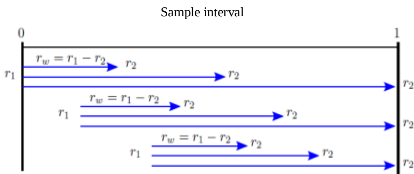
شکل ۱. فرآیند آزمون قوی سوپریمم دیکی - فولر تعمیم‌یافته منبع: فیلیپس و همکاران (۲۰۱۵)
