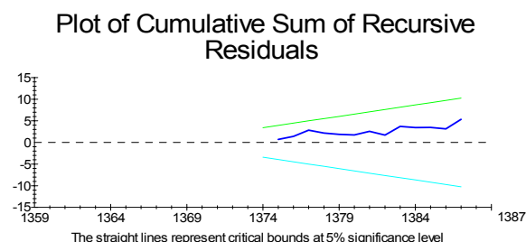
نمودار ۱. منحنی حاصل جمع انباشته پسماندها و مربعات پسماندها
