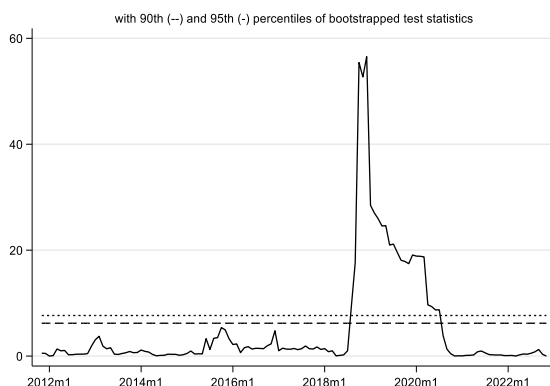
(ه) الگوریتم RE: نرخ ارز ← بازده شاخص کل علیت گرنجر (و) الگوریتم RO: نرخ ارز ← بازده شاخص کل علیت گرنجر
