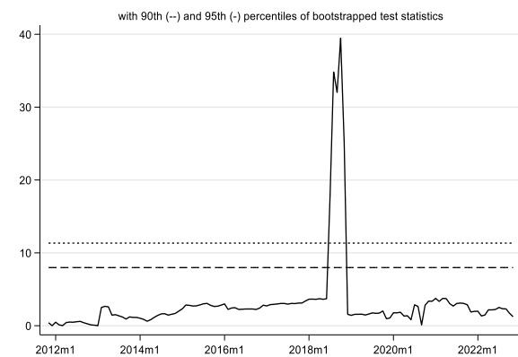
(ج) الگوریتم RE: بازده شاخص کل ← علیت گرنجر ← نرخ ارز (د) الگوریتم FE: نرخ ارز ← علیت گرنجر ← بازده شاخص کل
