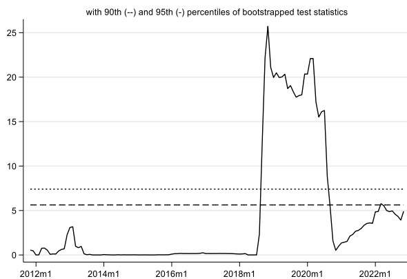
(الف) الگوریتم FE: بازده شاخص کل ← علیت گرنجر ← نرخ ارز (ب) الگوریتم RO: بازده شاخص کل ← علیت گرنجر ← نرخ ارز
