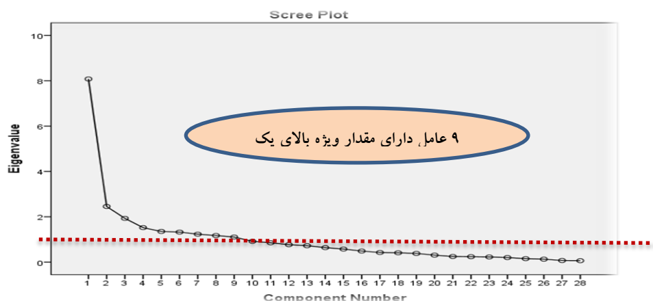
شکل ۱: نمودار سنگ‌ریزه (اسکری پلات) ۱ (مأخذ: یافته‌های تحقیق)
